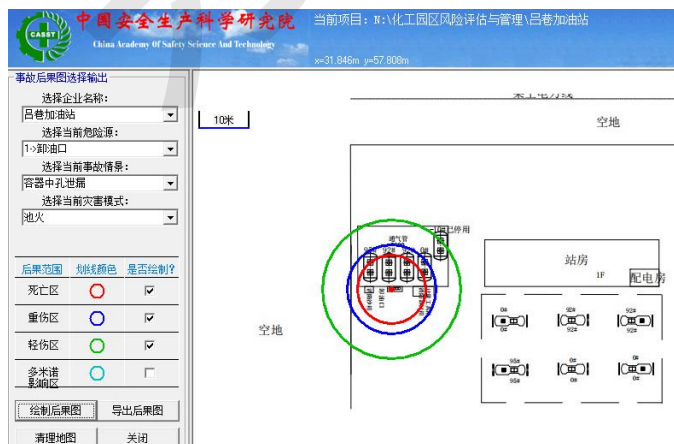
图 5-1 卸车点池火灾模拟图
